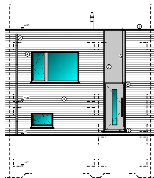
FACADE AVANT
