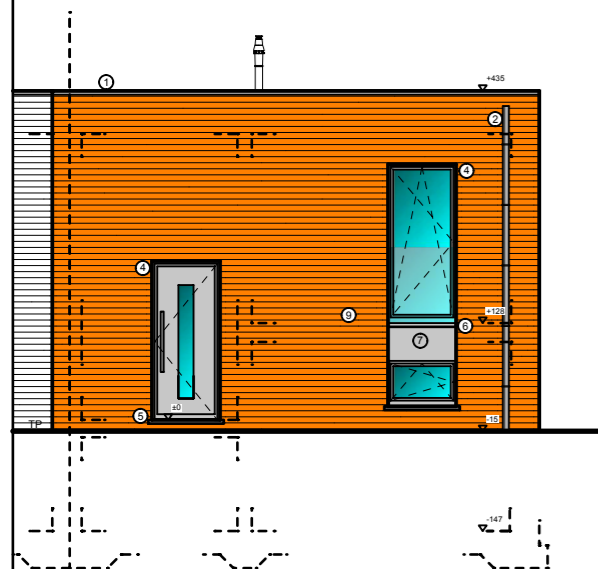
FACADE AVANT
